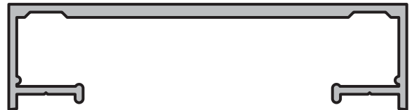
MARCO - PUERTA VAIVEN Perfil: 24 Peso: 0,730 Kg/m Matriz: M0693
