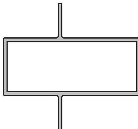
TUBO RECTANGULAR CON DOS ALETAS DE 60 x 25 x 1,6 mm. Perfil: 3994 Peso: 0,834 Kg/m
