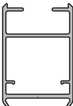
PARANTE POSTIGON DE ABRIR PARA 5800
