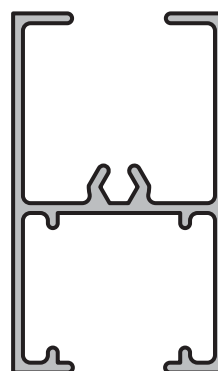
TRAVESAÑO POSTIGON DE ABRIR PARA 5800
