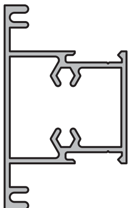
TRAVESAÑO ANGOSTO
