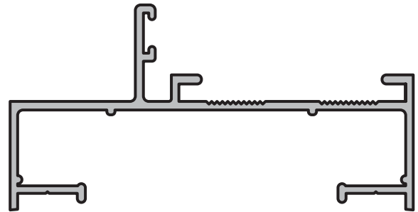
MARCO Perfil: 5362 Peso: 0,745 Kg/m
