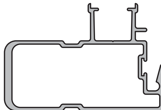
PARANTE CENTRAL REFORZADO - PUERTA CORREDIZA Perfil: 204 Peso: 1,112 Kg/m Matriz: M2632
