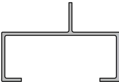
CANAL CON UNA ALETA DE 60 x 25 x 1,6 mm. Perfil: 3993 Peso: 0,594 Kg/m
