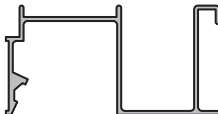
GUÍA CORTINA DE ENROLLAR Perfil: 920 Peso: 0,456 Kg/m Matriz: M2355
