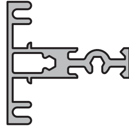
TRAVESANO VIDRIO REPARTIDO Perfil: M-2665 Peso: 0,562 Kg/m Matriz: M2665
