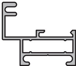
POSTIGO Perfil: M-2562 Peso: 0,419 Kg/m Matriz: M2562
