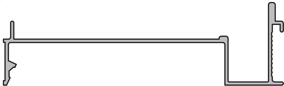
GUÍA DE CORTINA BARRIOS Perfil: 21 Peso: 0,926 Kg/m Matriz: M0690
