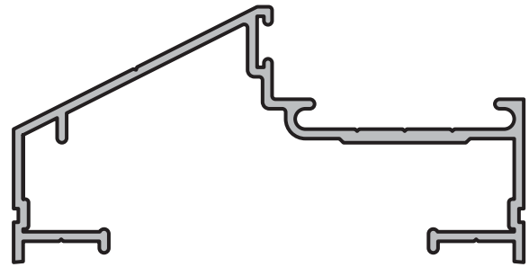
MARCO Perfil: M-2473 Peso: 0,724 Kg/m Matriz: M2473
