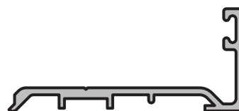
TAPACANTO CENTRAL HOJA Perfil: 214 Peso: 0,275 Kg/m Matriz: M2702
