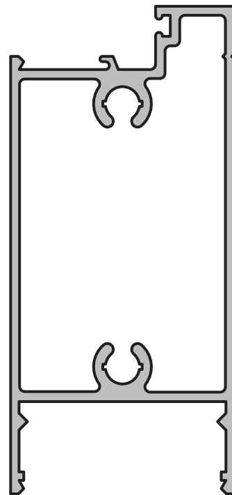
ZOCALO Perfil: 5624 Peso: 1,569 Kg/m
