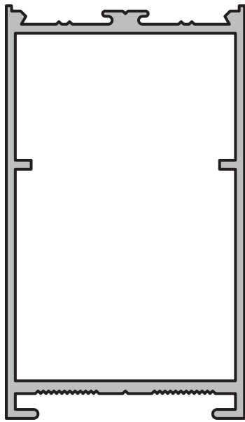
HOJA Perfil: 5616 Peso: 1,288 Kg/m
