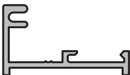
PORTACONTRAVIDRIO UNIVERSAL SIMPLE Perfil: 52 Peso: 0,300 Kg/m Matriz: M0947
