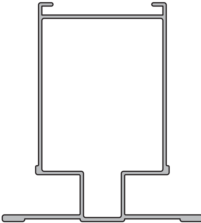
GUÍA CENTRAL - CORTINA BARRIOS Perfil: 131 Peso: 1,723 Kg/m Matriz: M1852
