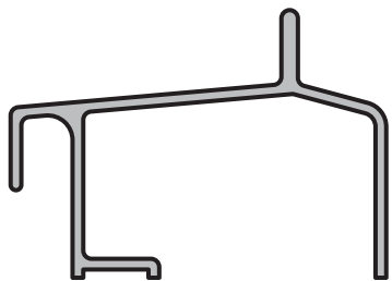
UMBRAL SANITARIO Perfil: 6926 Peso: 0,419 Kg/m
