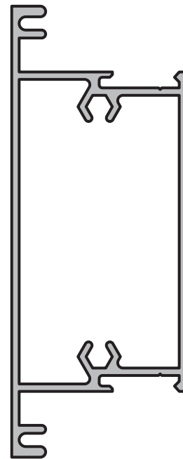
TRAVESANO ANCHO Perfil: M-2212 Peso: 1,010 Kg/m Matriz: M2212
