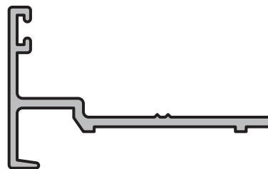
DOBLE CONTACTO Perfil: 5622 Peso: 0,418 Kg/m
