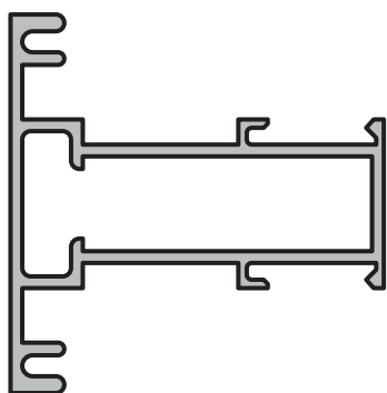
TRAVESAÑO PARA VIDRIO PARTIDO Perfil: 209 Peso: 0,718 Kg/m Matriz: M2697
