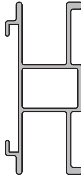
GUÍA CENTRAL - CORTINA COMUN Perfil: 130 Peso: 1,053 Kg/m Matriz: M1851
