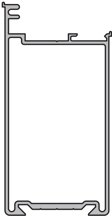
BATIANTE DE HOJA Perfil: 213 Peso: 1,226 Kg/m Matriz: M2701
