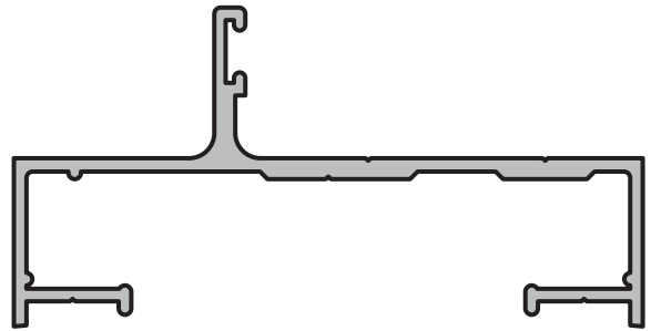
MARCO Perfil: 10 Peso: 0,788 Kg/m Matriz: M0676
