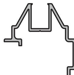
BASTIDOR VIDRIO REPARTIDO PAÑO FIJO
