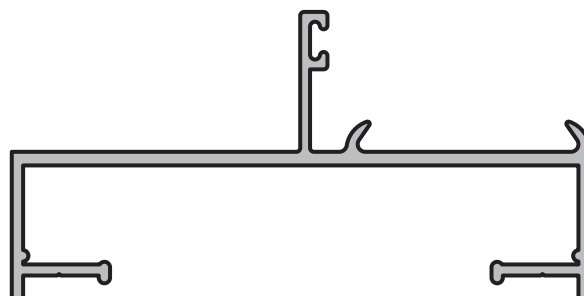
MARCO
