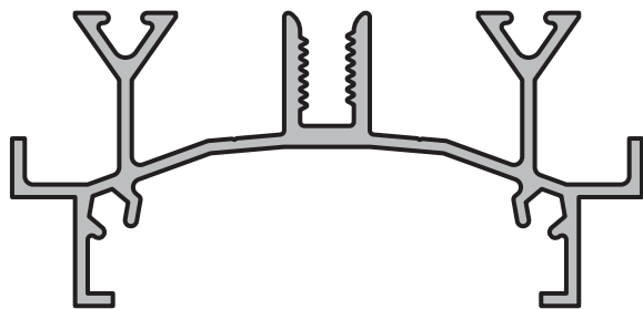
LARGUERO Perfil: 85 Peso: 1,013 Kg/m Matriz: M2769
